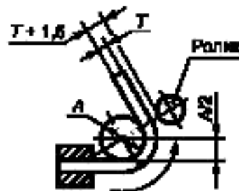
Конструкция с обкаткой роликом
