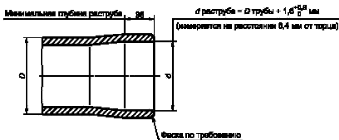
Рисунок 2 — Раструбный конец для соединения труб между собой
