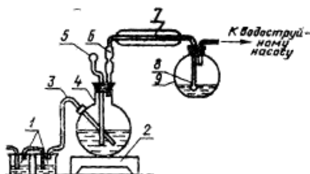
1—стаканки, заполненные водой и серной кислотой; 2—электроплитка; 3—стеклянная трубка диаметром 6—7 мм; 4—двухгорловая колба вместимостью 1 дм 3 ; 5—воронка; 6—кварцевый дефлегматор; 7—кварцевый холодильник; 8—кварцевый барботер; 9—колба приемника дистиллята
