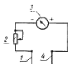
1—вольтовый электрод (проволока длиной 50 мм и диаметром 1—2 мм или спираль из нее); 2—переменный сопротивление на 25—50 кОм; 3—милливольтметр типа МПП 254 или милливольт-микромперметр типов М-95, М-193/2 или другого типа; 4—вольфрамовый электрод (проволока диаметром 0,5—1,0 мм или спираль из нее)
