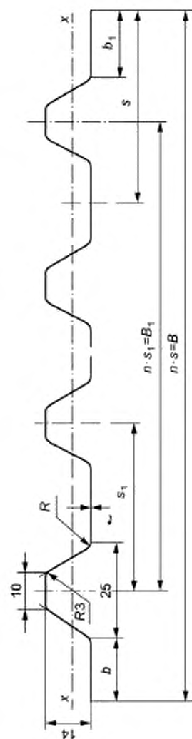
Рисунок 3 — Профили типа А высотой 14 мм
