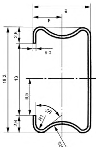
Рисунок 10 — Профили типа СА высотой 8 мм
