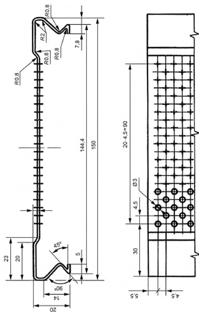
Рисунок 9 — Профили типа СА высотой 20 мм
