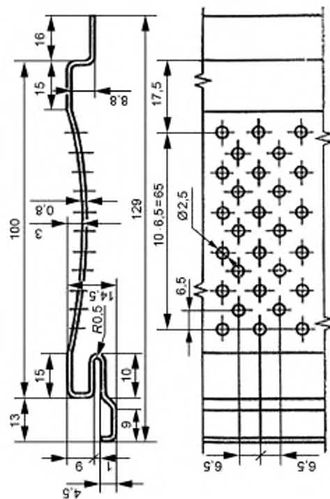
Рисунок 12 — Профили типа СА высотой 15 мм
