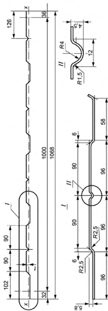
Рисунок 1 — Профили типа А высотой 6 мм
