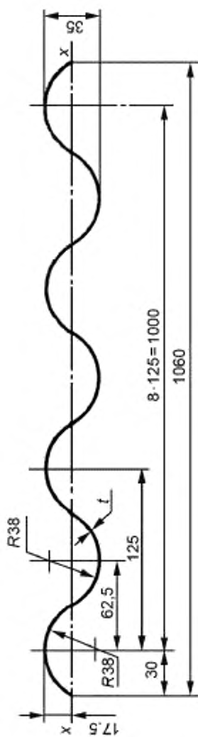
Рисунок 6 — Профили типа А высотой 35 мм
