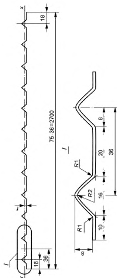
Рисунок 2 — Профили типа А высотой 8 мм
