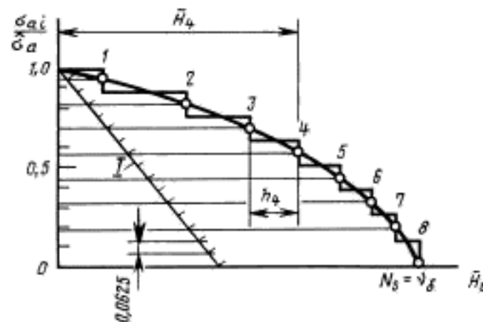
Линейное разбиение спектра нагружения на 8 ступеней
