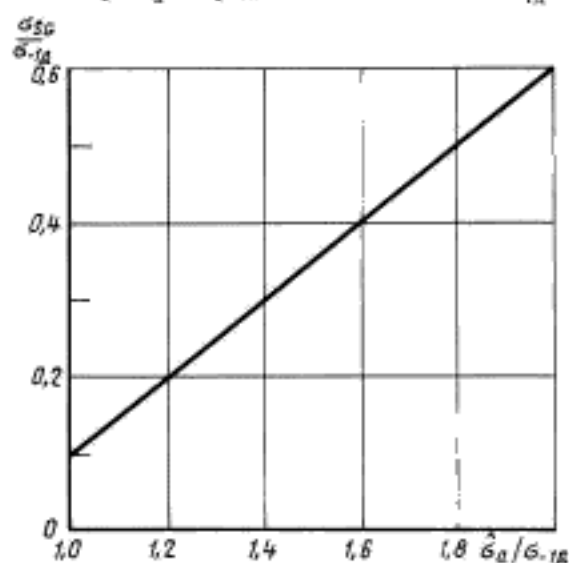
Значения повреждающих амплитуд \sigma_{SG} в зависимости от максимальной амплитуды спектра \hat{\sigma}_d и предела выносливости \sigma_{-1d}
