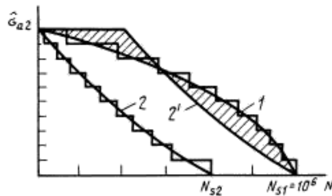
1 — спектр 1; 2 — спектр 2; 2' — спектр 2, расширенный до объема спектра N_{s1} = 10^6 ; — отличие форм обоих спектров
